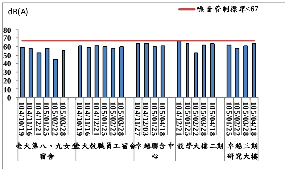
圖 2.3-4 營建噪音 L_{eq} 歷次監測結果趨勢圖
