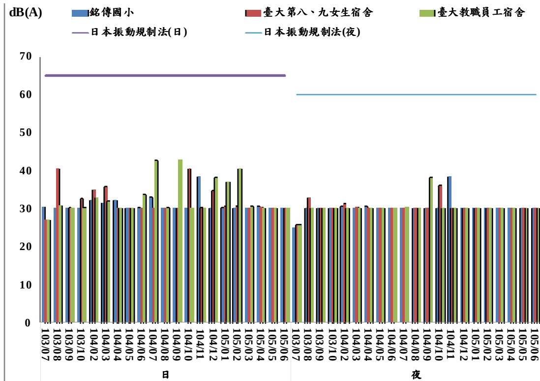
圖 2.3-2 振動歷次監測結果趨勢圖 (1/2)
