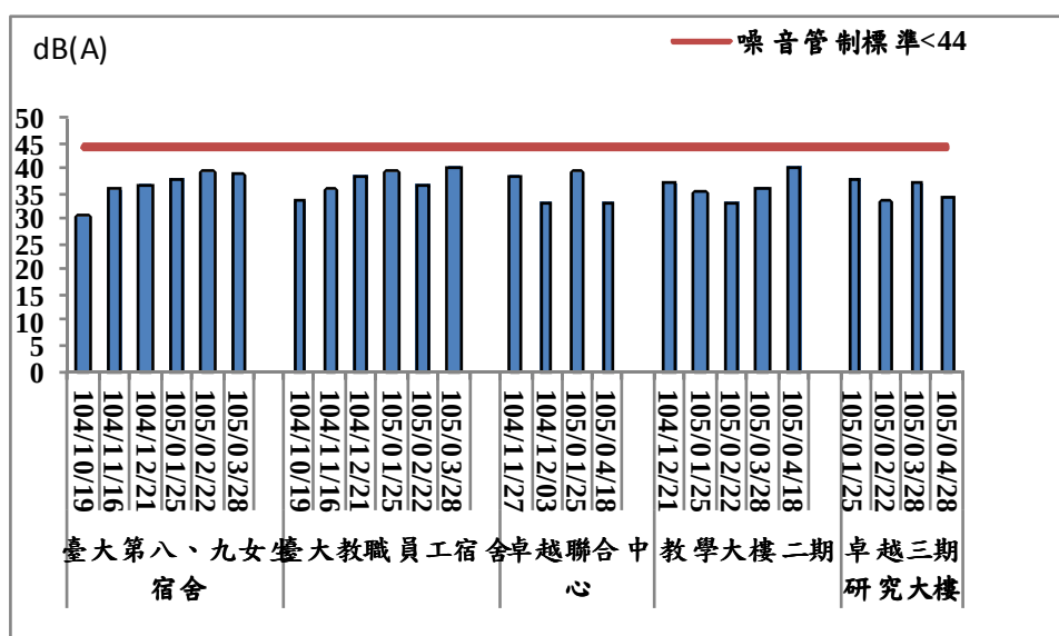
圖2.3-3 營建噪音 L_{eq,LF} 歷次監測結果趨勢圖
