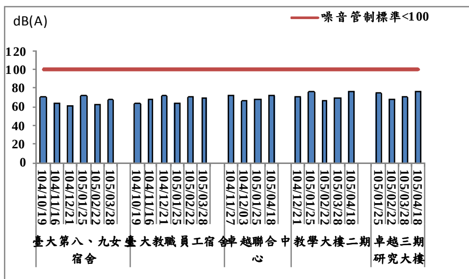
圖 2.3-5 營建噪音 L_{max} 歷次監測結果趨勢圖
