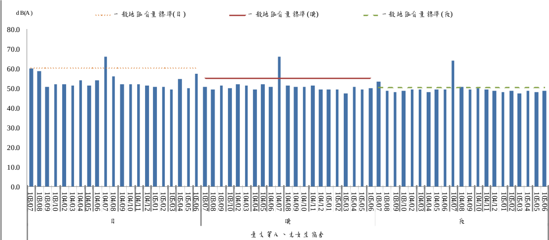
圖 2.3-1 噪音歷次監測結果趨勢圖 (2/6)
