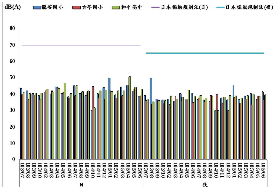
圖 2.3-2 振動歷次監測結果趨勢圖 (2/2)
