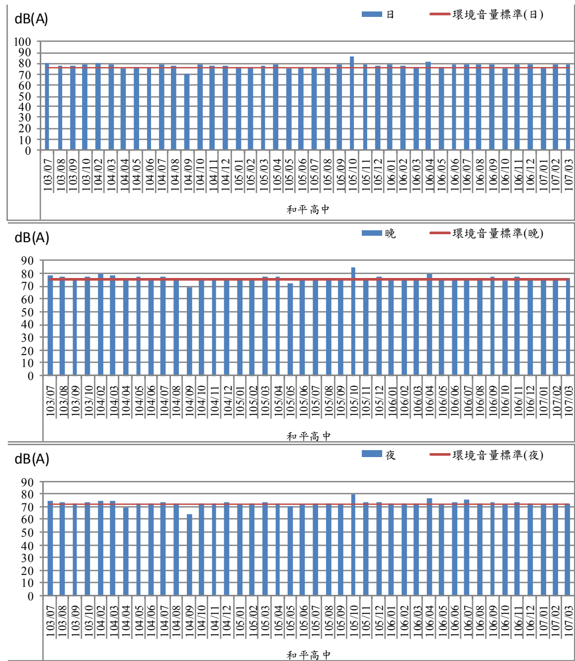
圖2.3-6 噪音歷次監測結果趨勢圖—和平高中
