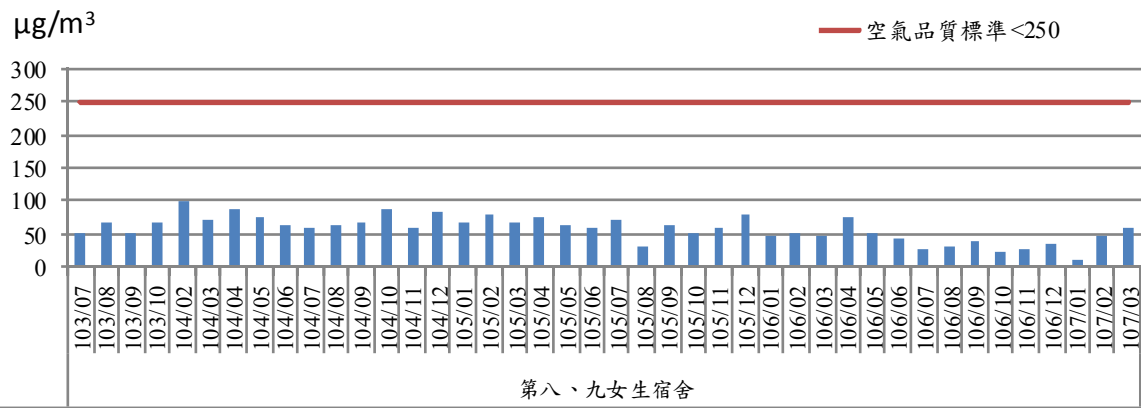
圖2.1-1 總懸浮微粒二十四小時值歷次監測結果趨勢圖(4/4)
