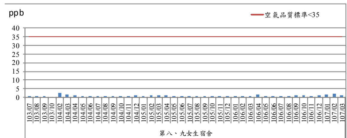
圖2.1-8 一氧化碳最高小時平均值歷次監測結果趨勢圖(4/4)
