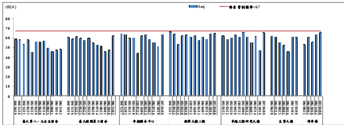
圖2.3-4 營建噪音 L_{eq} 歷次監測結果趨勢圖
