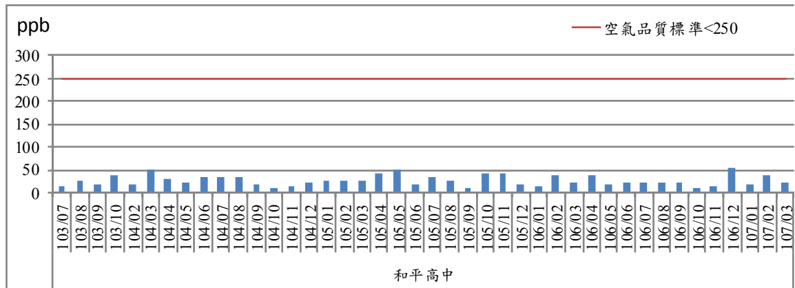
圖2.1-5 二氧化氮最高小時平均值歷次監測結果趨勢圖(1/4)
