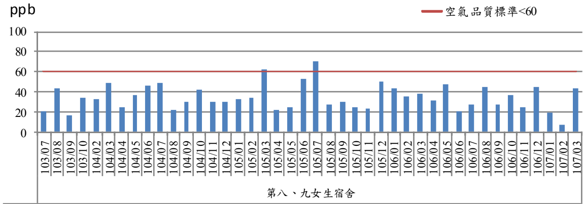
圖2.1-4 臭氧八小時平均值歷次監測結果趨勢圖(4/4)
