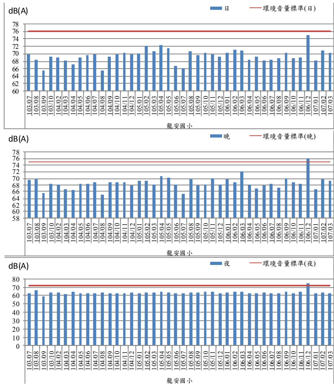
圖2.3-4 噪音歷次監測結果趨勢圖－龍安國小
