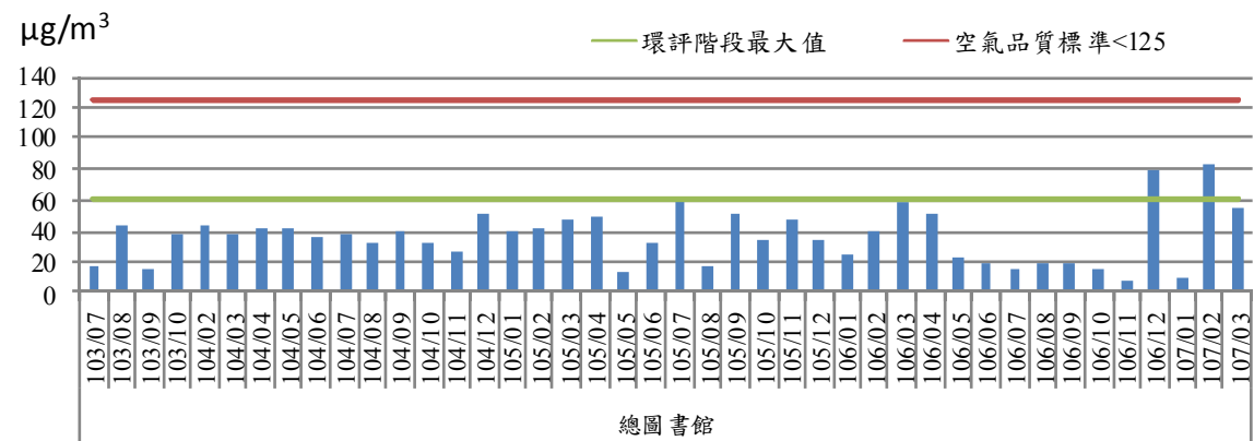
圖2.1-2 懸浮微粒日平均值歷次監測結果趨勢圖(3/4)
