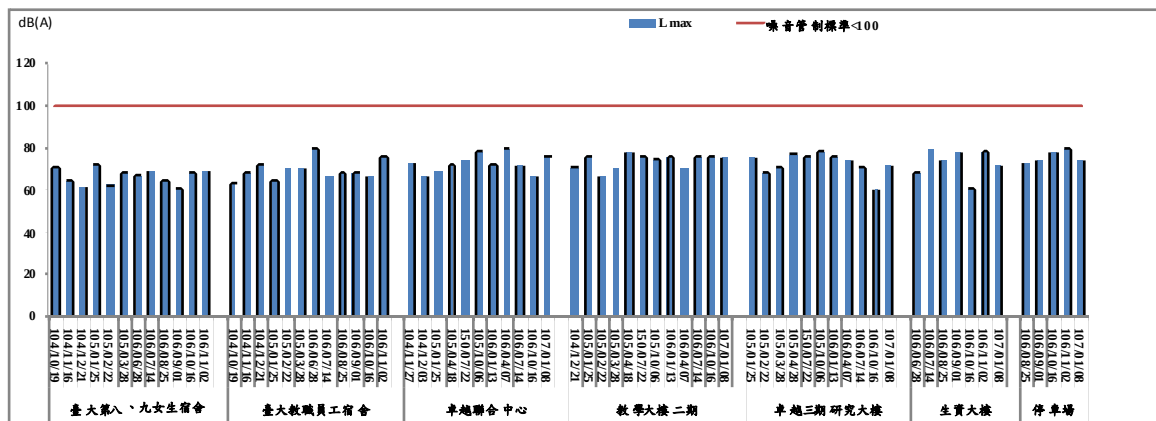
圖2.3-5 營建噪音 L_{max} 歷次監測結果趨勢圖
