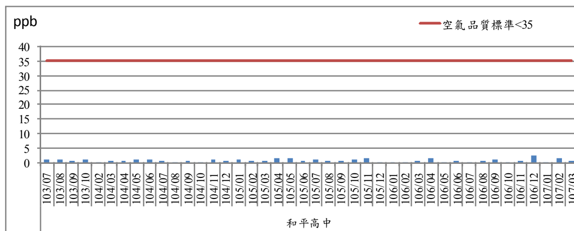
圖2.1-8 一氧化碳最高小時平均值歷次監測結果趨勢圖(1/4)
