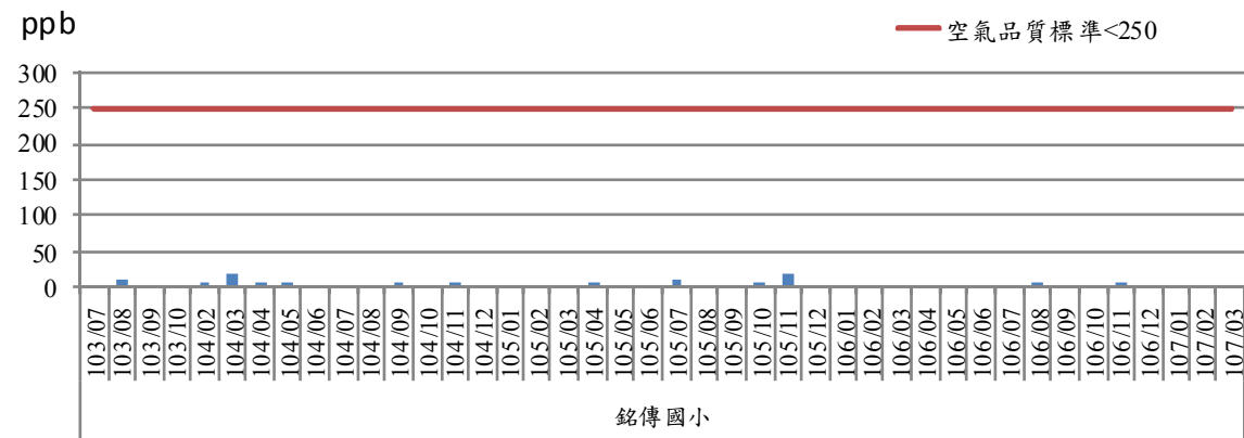
圖2.1-6 二氧化硫最高小時平均值歷次監測結果趨勢圖(2/4)
