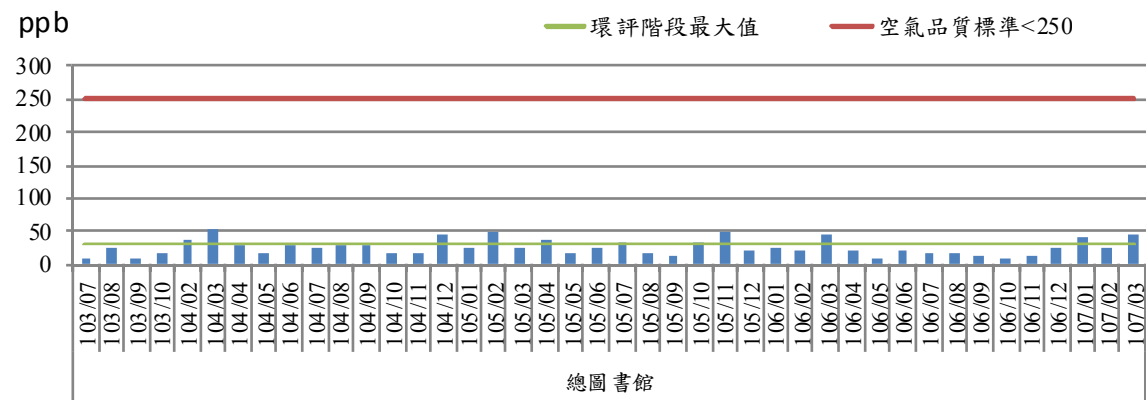
圖2.1-5 二氧化氮最高小時平均值歷次監測結果趨勢圖(3/4)
