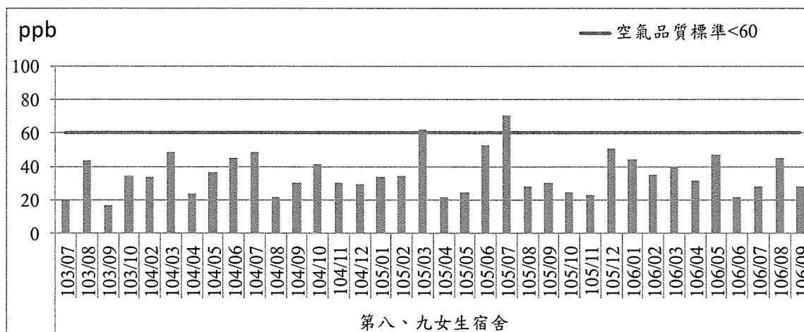
圖2.1-4 臭氧八小時平均值歷次監測結果趨勢圖(4/4)
