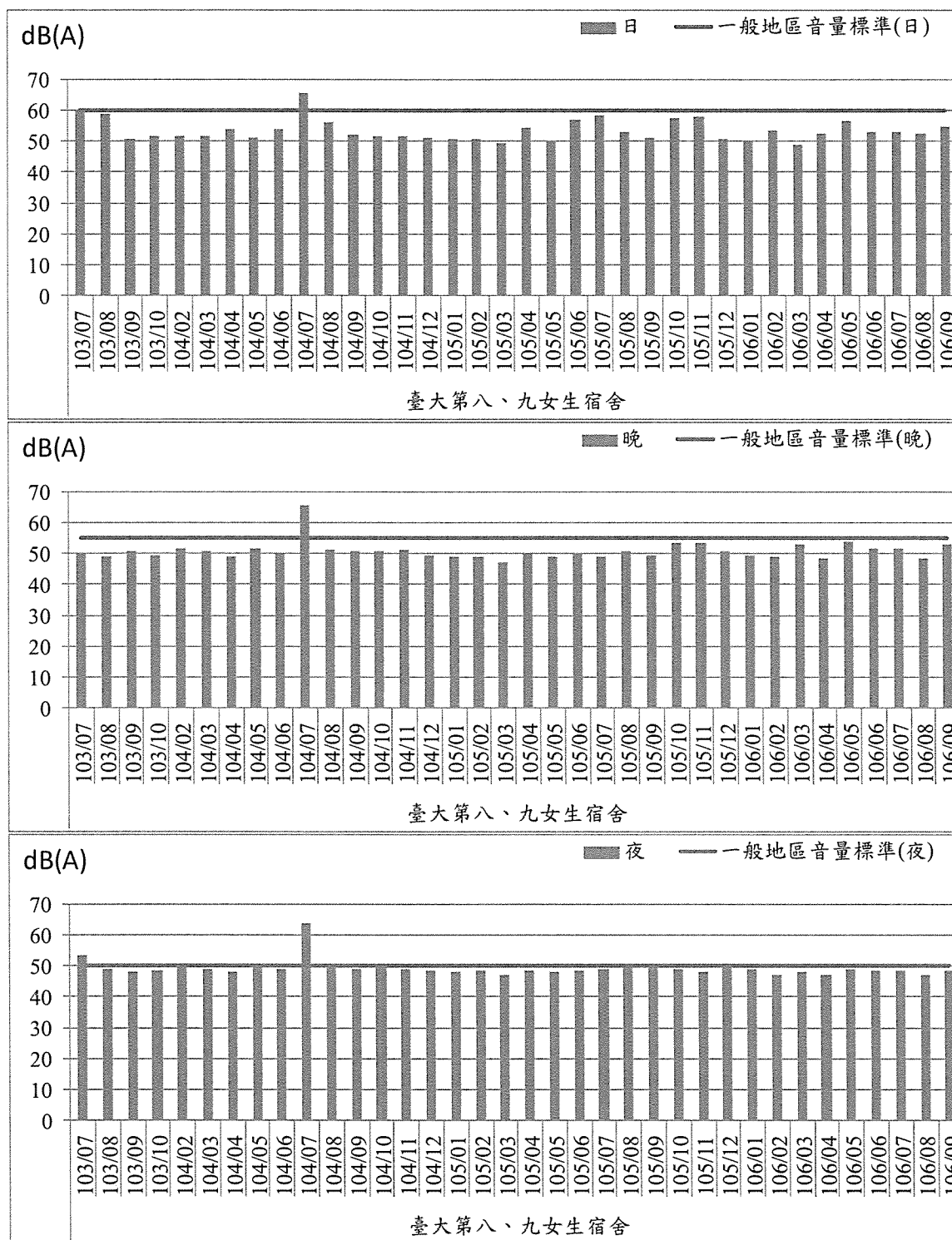
圖2.3-2 噪音歷次監測結果趨勢圖－臺大第八九女生宿舍
