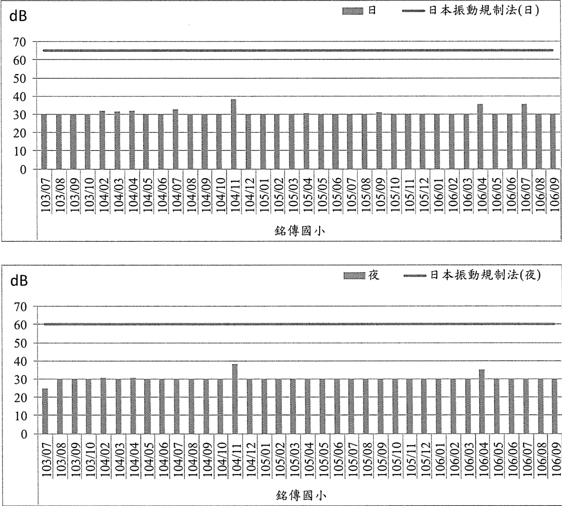
圖2.3-7 振動歷次監測結果趨勢圖－銘傳國小
