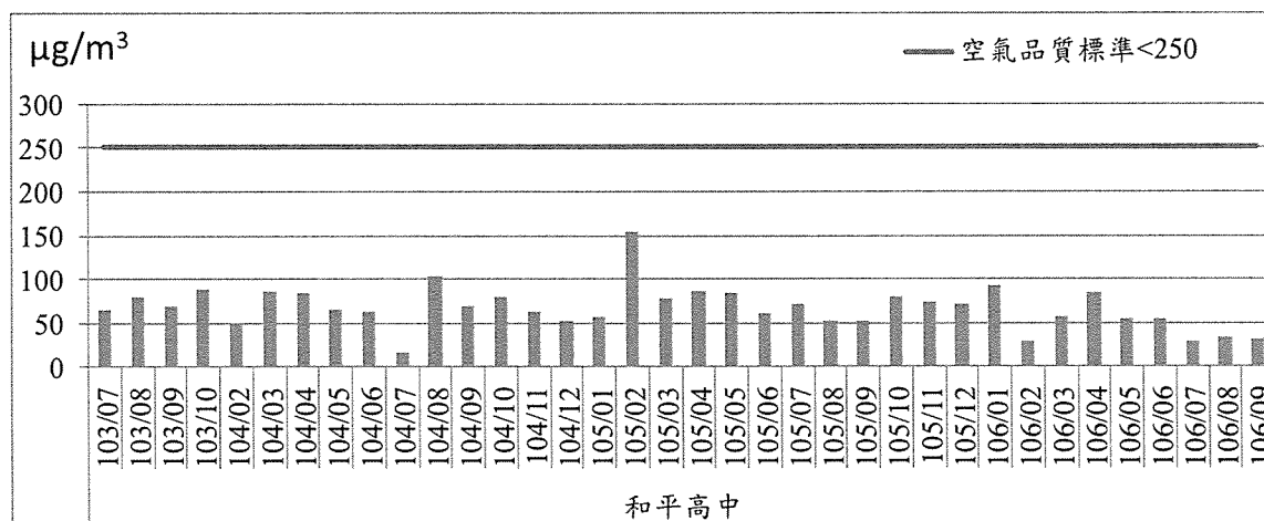
圖2.1-1 總懸浮微粒二十四小時值歷次監測結果趨勢圖(1/4)
