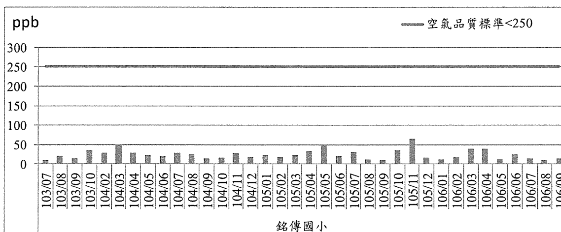
圖2.1-5 二氧化氮最高小時平均值歷次監測結果趨勢圖(2/4)
