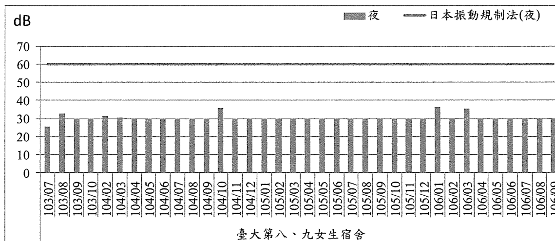
圖2.3-8 振動歷次監測結果趨勢圖－臺大第八九女生宿舍
