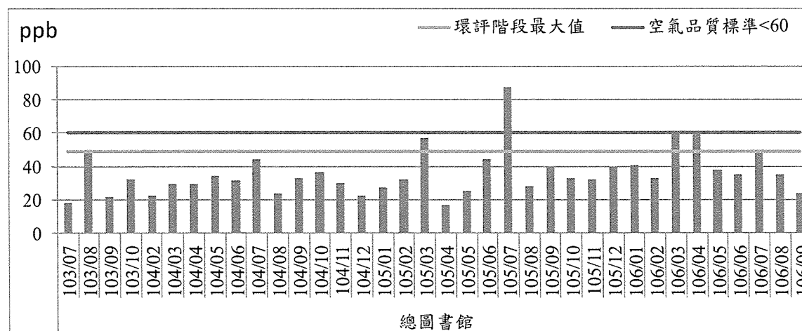
圖2.1-4 臭氧八小時平均值歷次監測結果趨勢圖(3/4)
