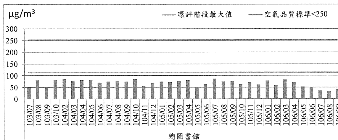
圖2.1-1 總懸浮微粒二十四小時值歷次監測結果趨勢圖(3/4)
