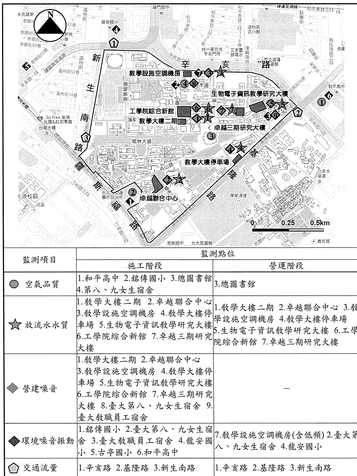
圖1.4-1 本計畫監測位置示意圖
