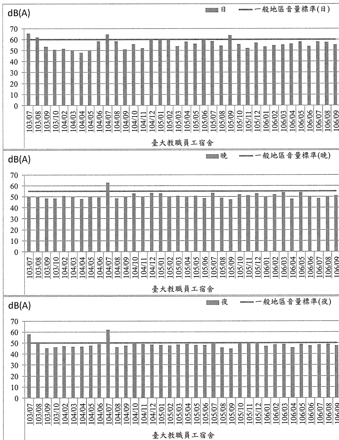
圖2.3-3 噪音歷次監測結果趨勢圖－臺大教職員工宿舍
