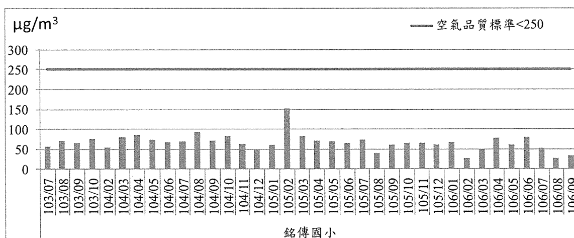
圖2.1-1 總懸浮微粒二十四小時值歷次監測結果趨勢圖(2/4)
