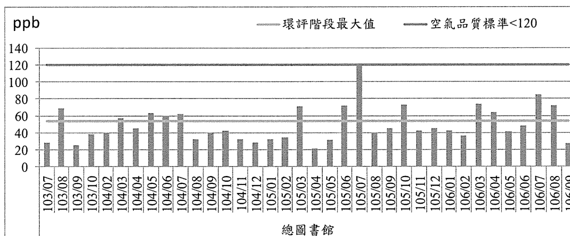
圖2.1-3 臭氧最高小時平均值歷次監測結果趨勢圖(3/4)
