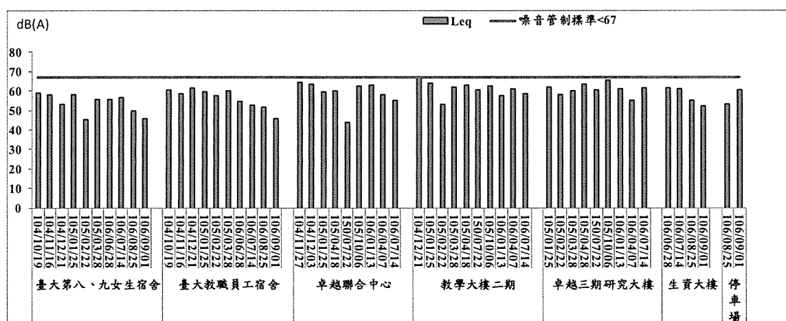
圖2.3-4 營建噪音 L_{eq} 歷次監測結果趨勢圖
