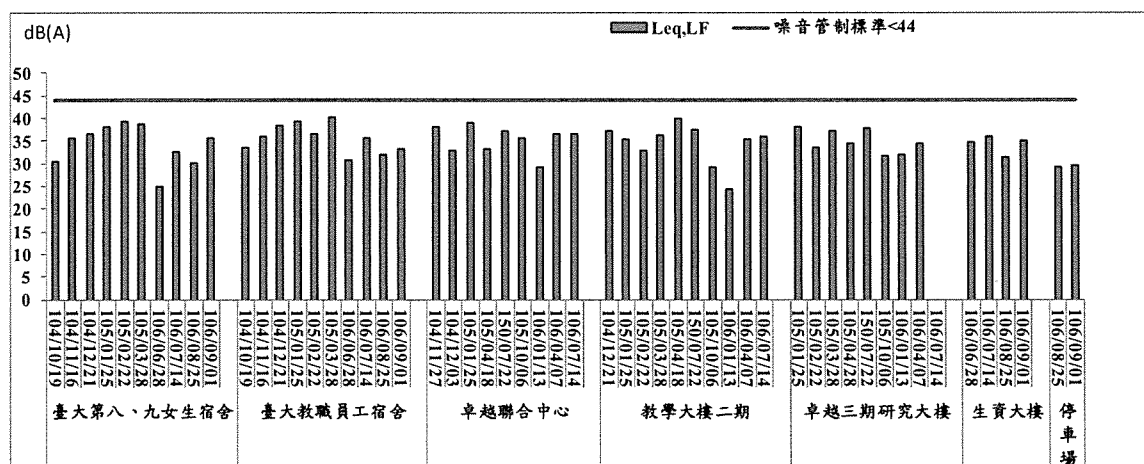
圖2.3-3 營建噪音 L_{eq,LF} 歷次監測結果趨勢圖
