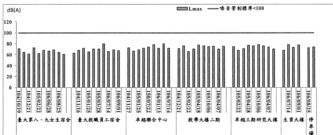
圖2.3-5 營建噪音 L_{max} 歷次監測結果趨勢圖
