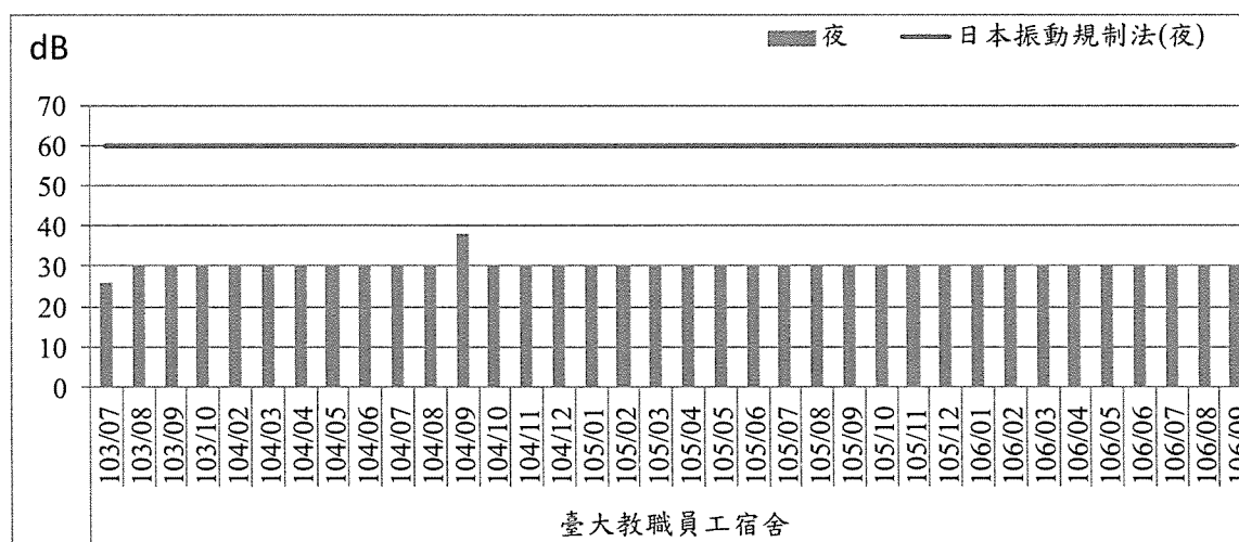
圖2.3-9 振動歷次監測結果趨勢圖－臺大教職員工宿舍
