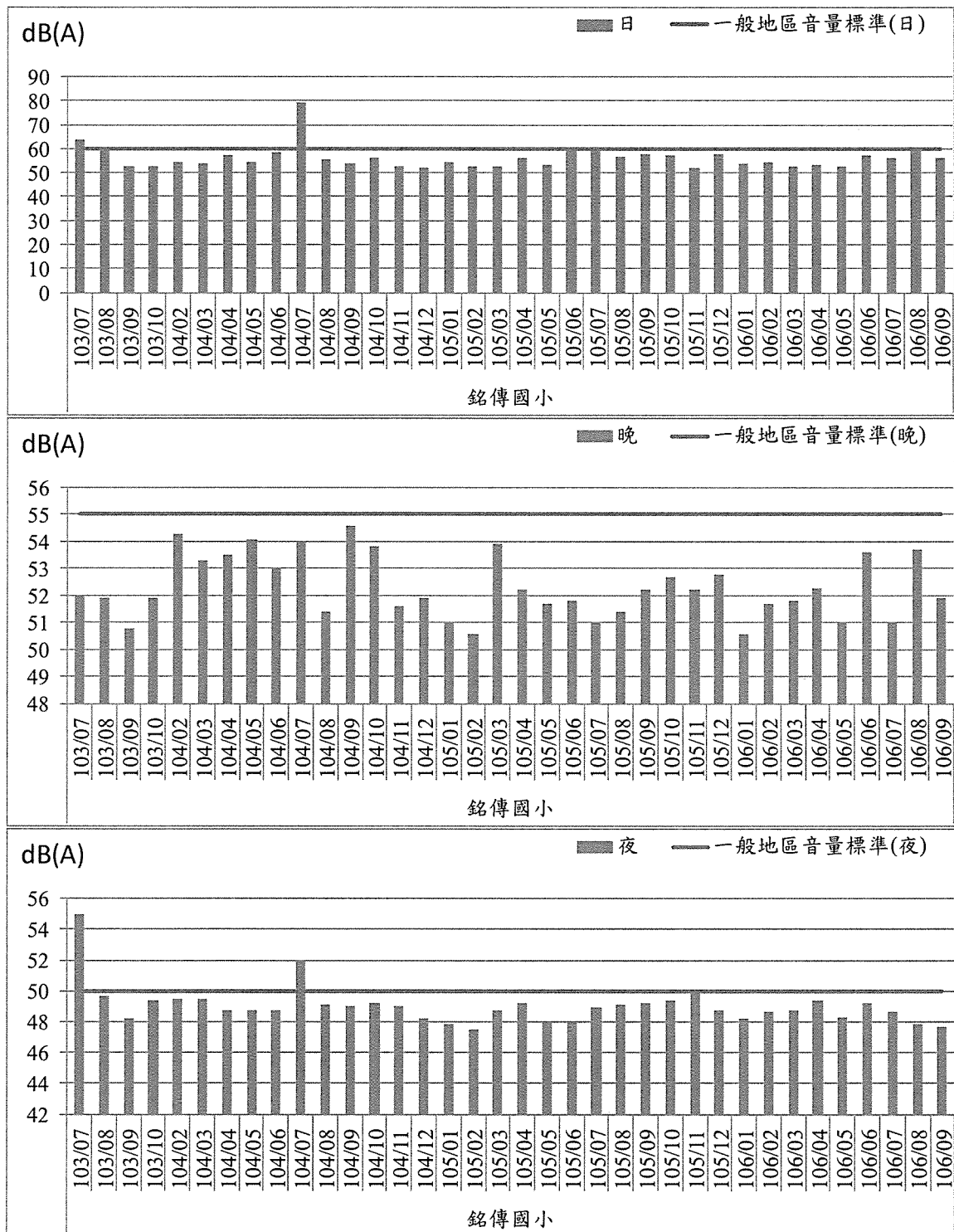
圖2.3-1 噪音歷次監測結果趨勢圖－銘傳國小
