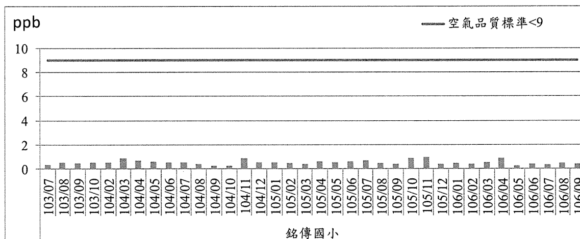
圖2.1-10 一氧化碳八小時平均值歷次監測結果趨勢圖(2/4)
