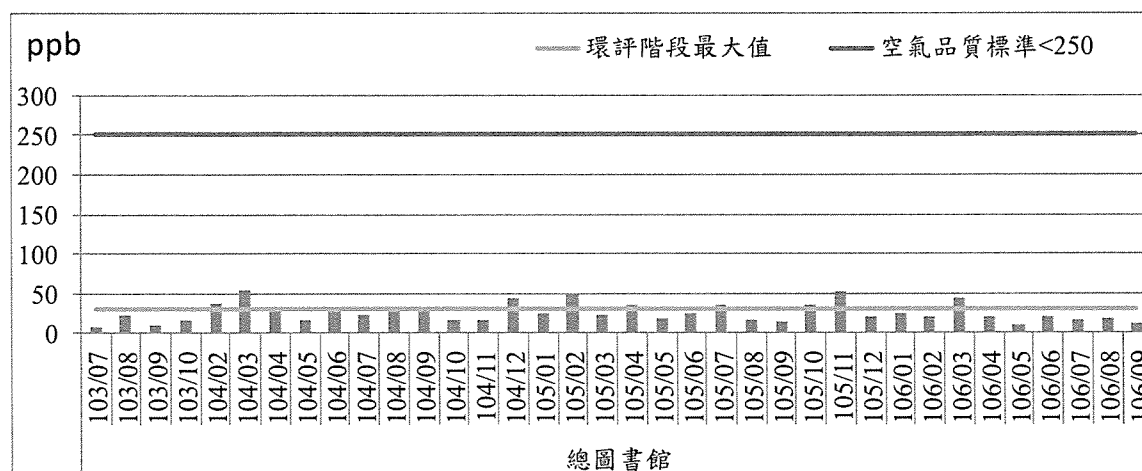
圖2.1-5 二氧化氮最高小時平均值歷次監測結果趨勢圖(3/4)
