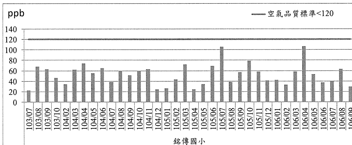
圖2.1-3 臭氧最高小時平均值歷次監測結果趨勢圖(2/4)
