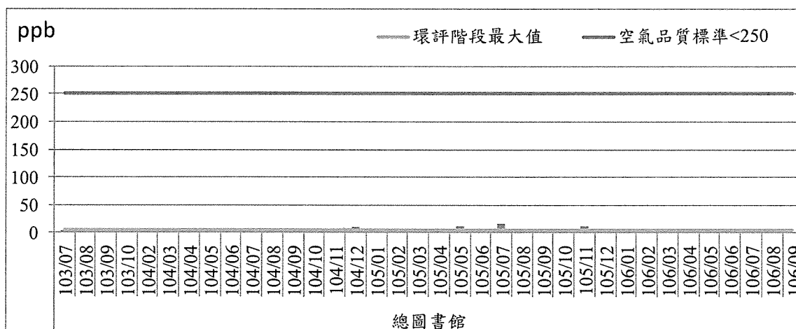
圖2.1-6 二氧化硫最高小時平均值歷次監測結果趨勢圖(3/4)
