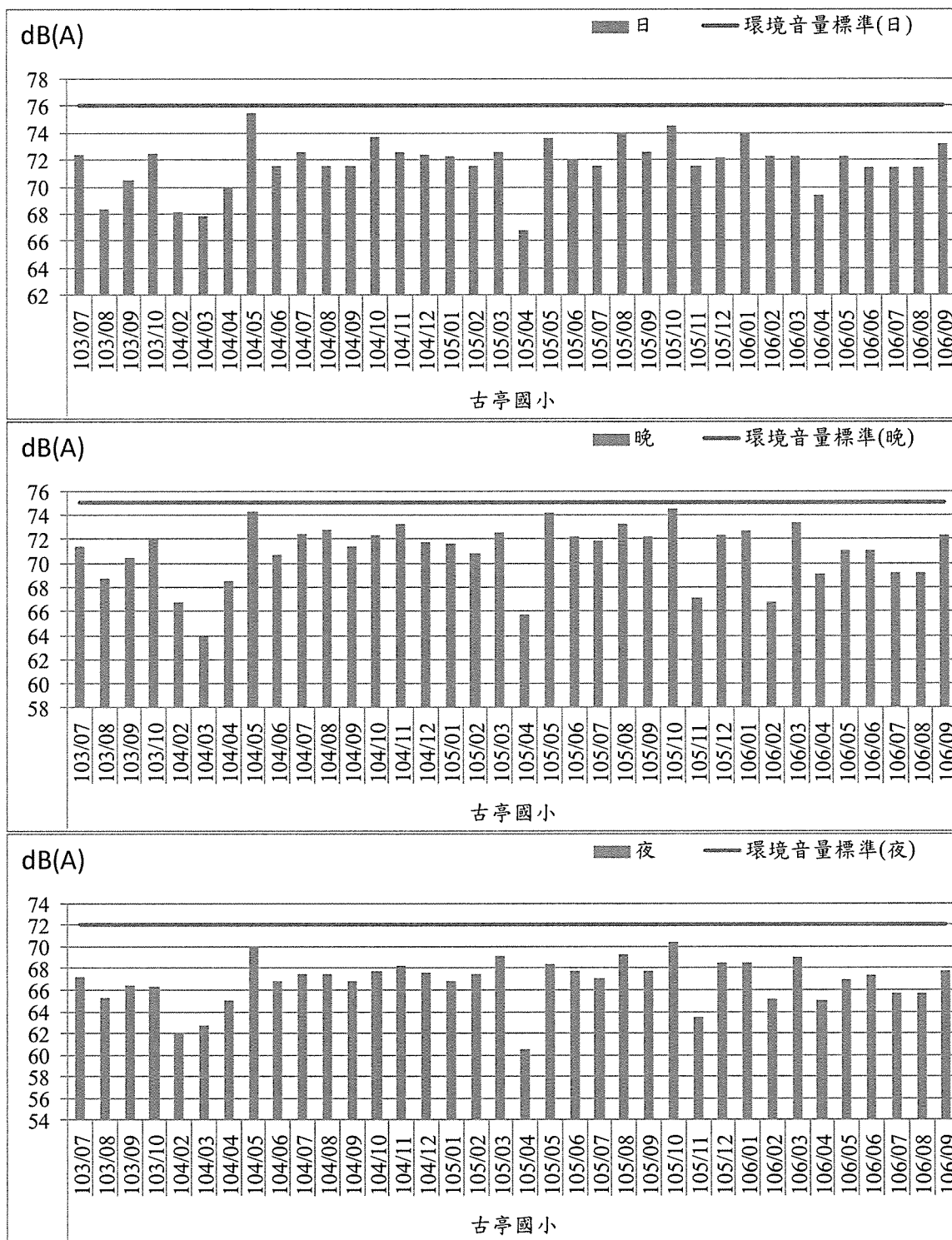
圖2.3-5 噪音歷次監測結果趨勢圖—古亭國小
