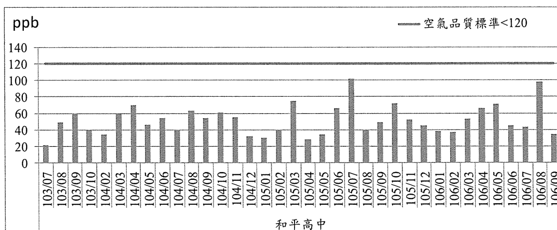
圖2.1-3 臭氧最高小時平均值歷次監測結果趨勢圖(1/4)
