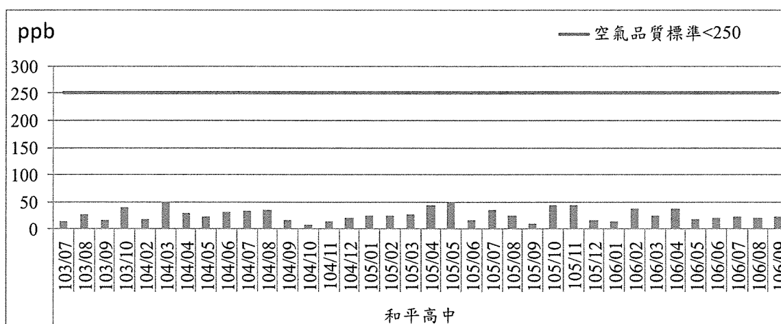
圖2.1-5 二氧化氮最高小時平均值歷次監測結果趨勢圖(1/4)
