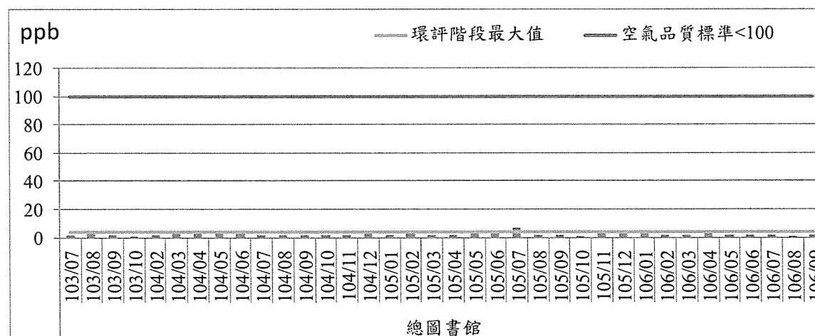
圖2.1-7 二氧化硫日平均值歷次監測結果趨勢圖(3/4)
