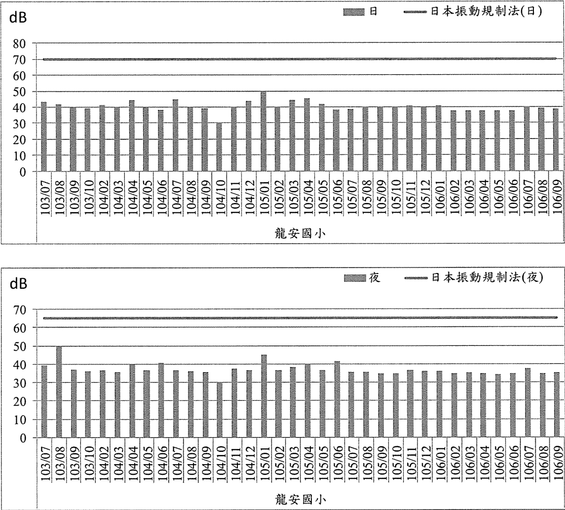
圖2.3-10 振動歷次監測結果趨勢圖－龍安國小
