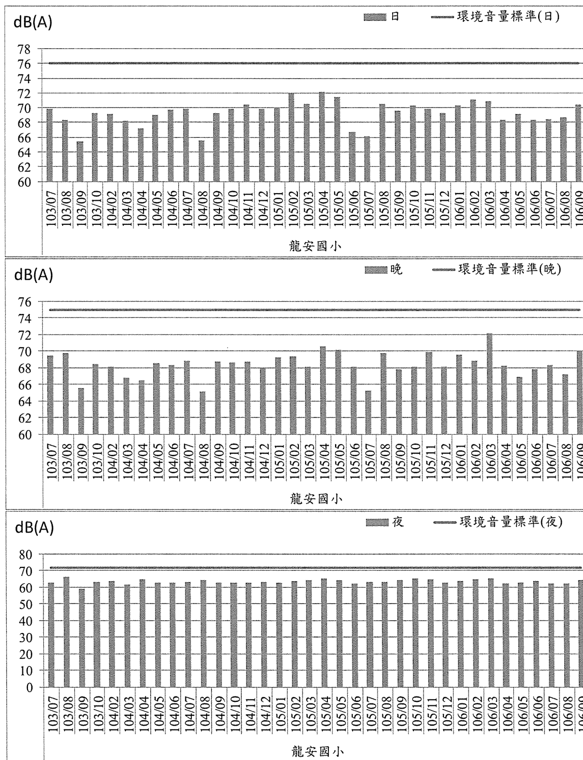
圖2.3-4 噪音歷次監測結果趨勢圖－龍安國小
