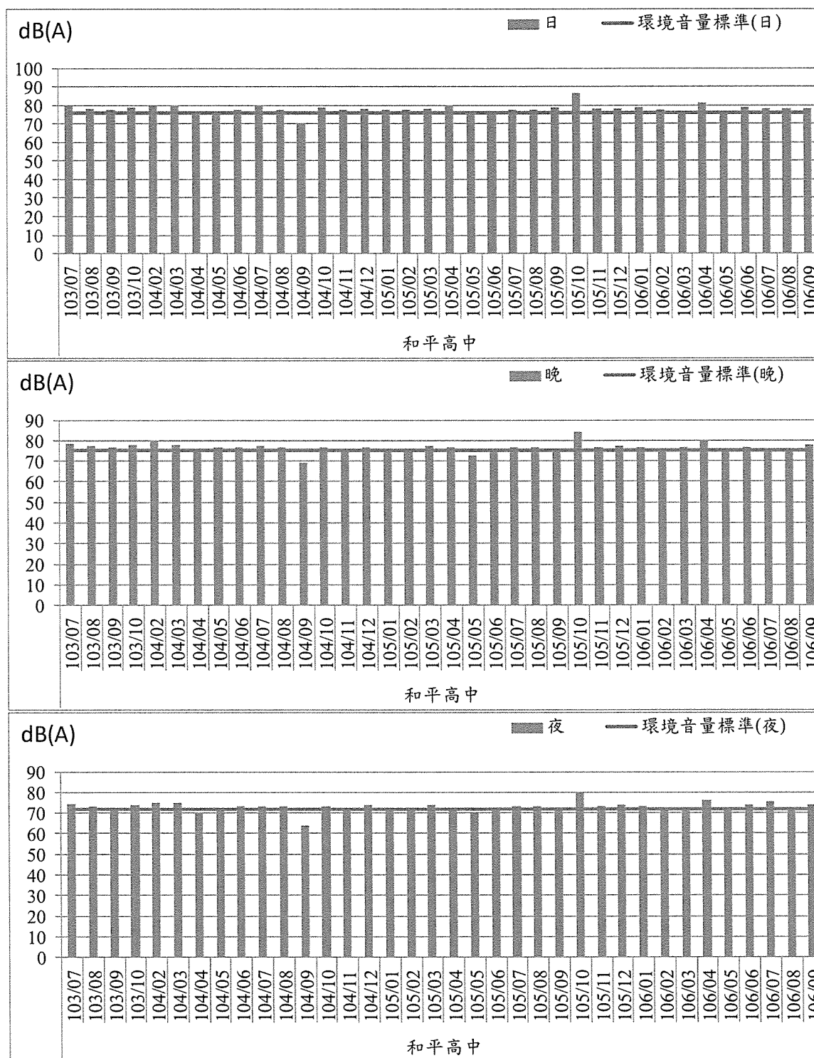
圖2.3-6 噪音歷次監測結果趨勢圖－和平高中
