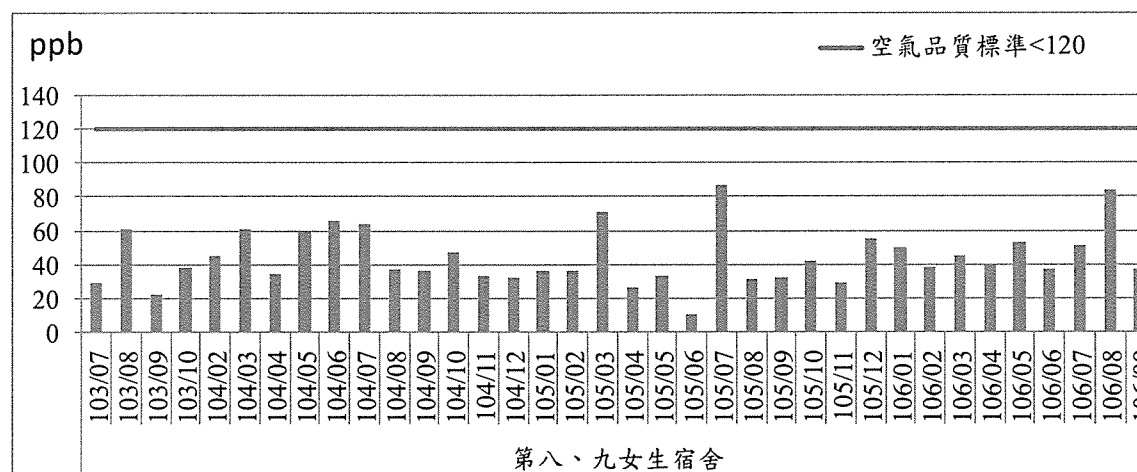
圖2.1-3 臭氧最高小時平均值歷次監測結果趨勢圖(4/4)
