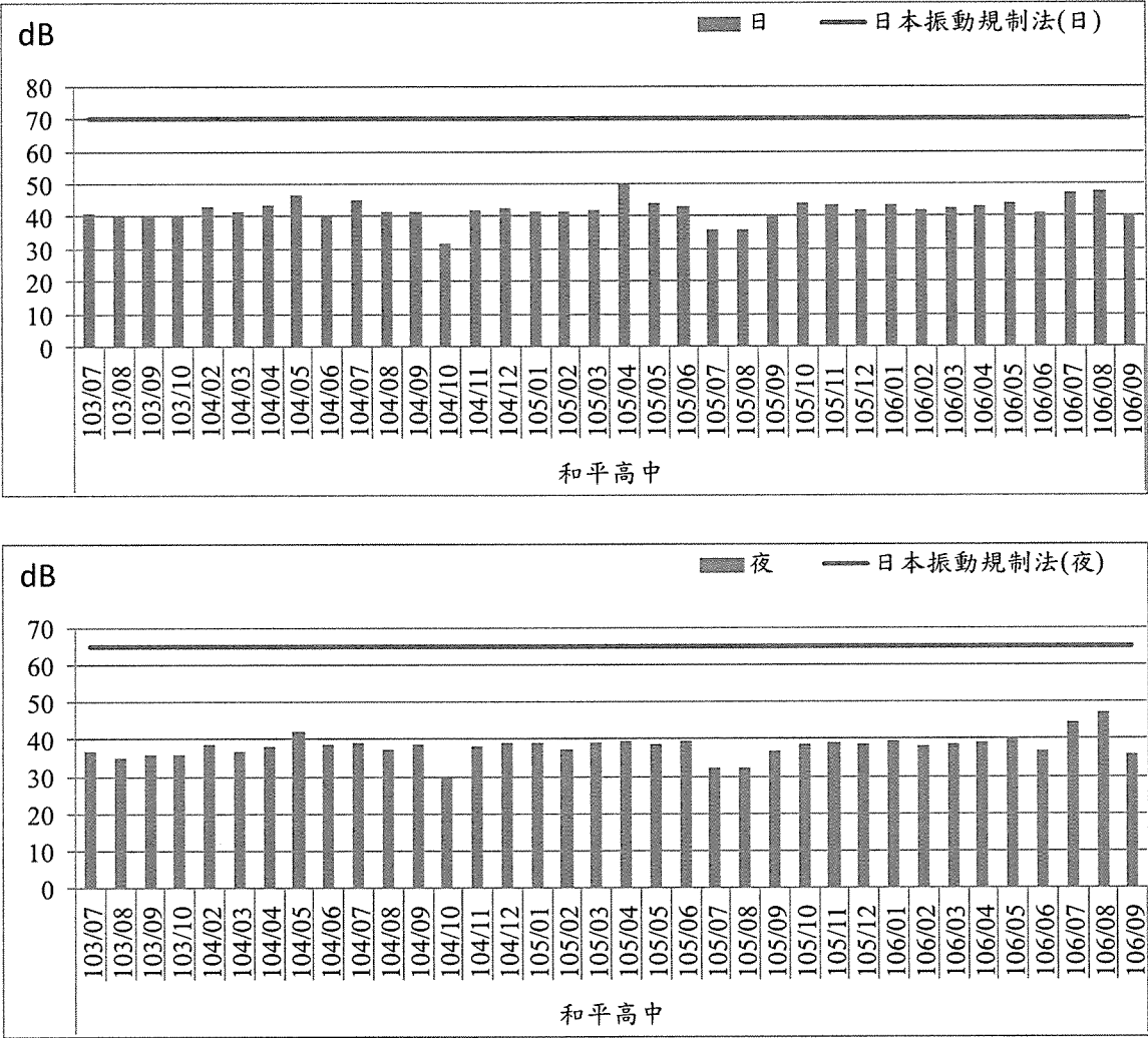
圖2.3-12 振動歷次監測結果趨勢圖－和平高中
