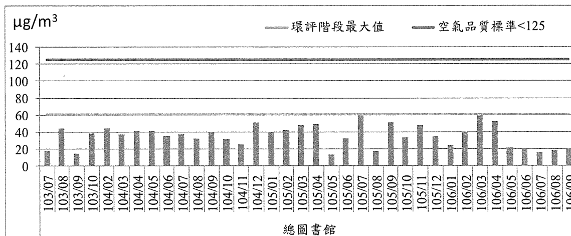
圖2.1-2 懸浮微粒日平均值歷次監測結果趨勢圖(3/4)
